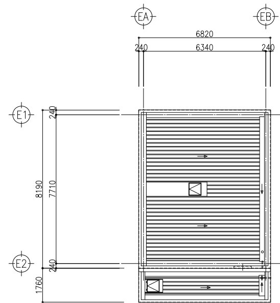
屋根伏図
