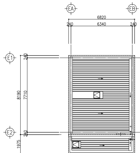
屋根伏図
