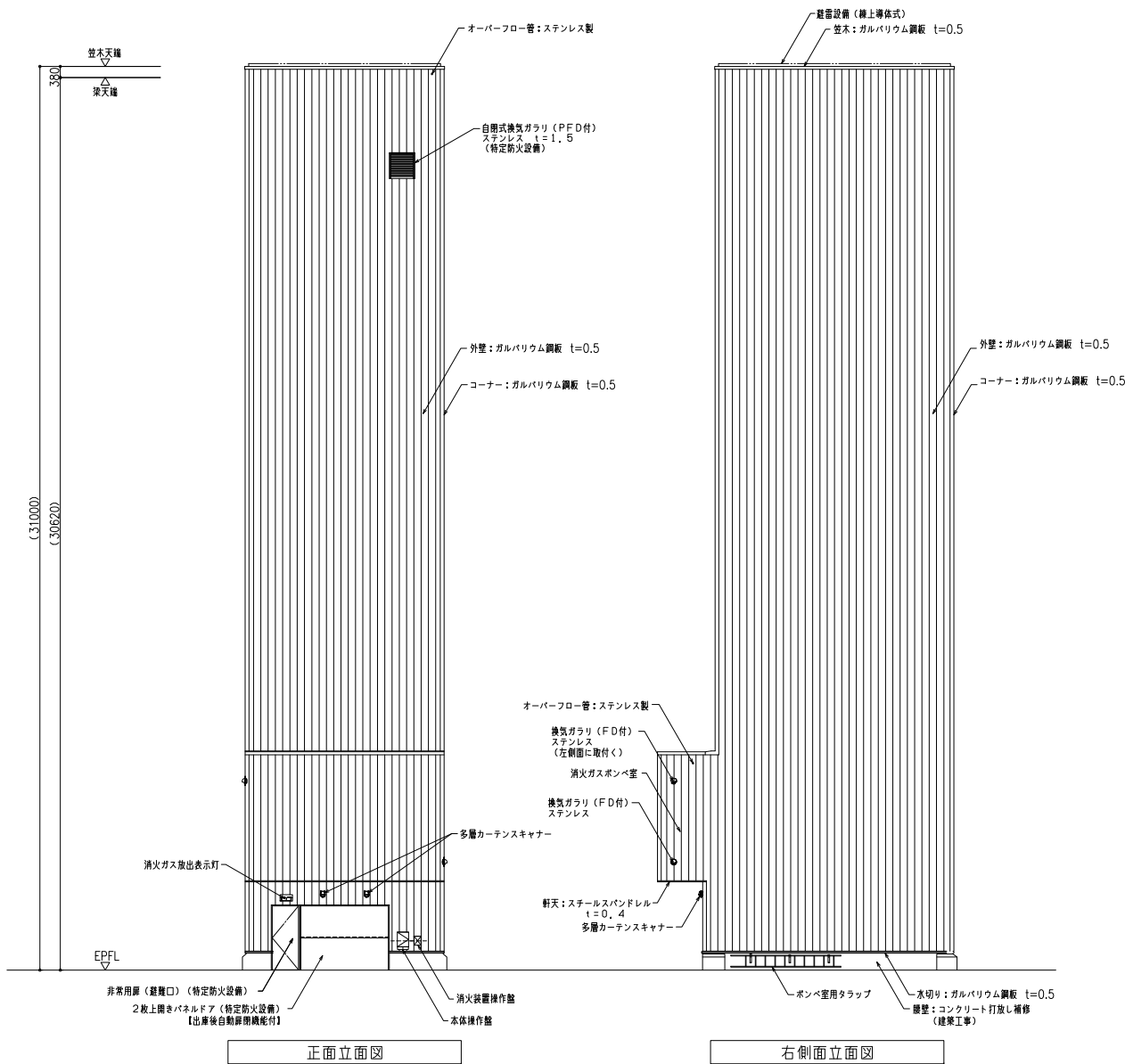
正面立面図
