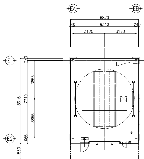
平面配置図
