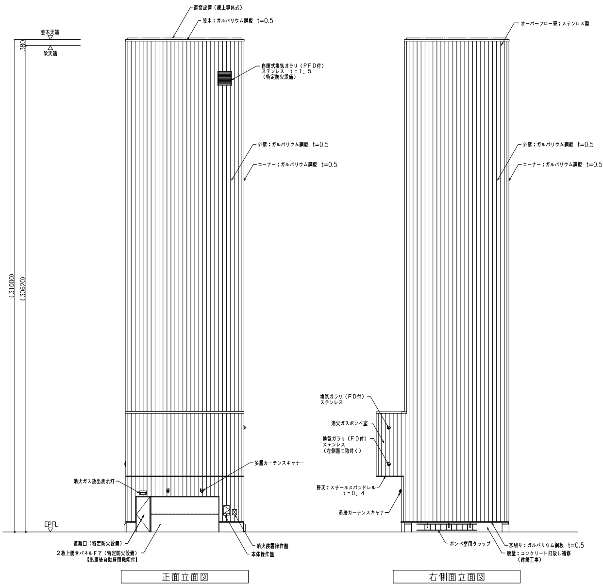
正面立面図
