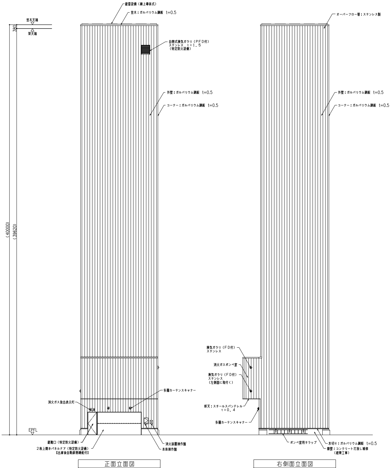
正面立面図
