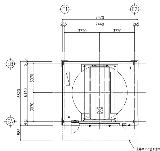
平面配置図
