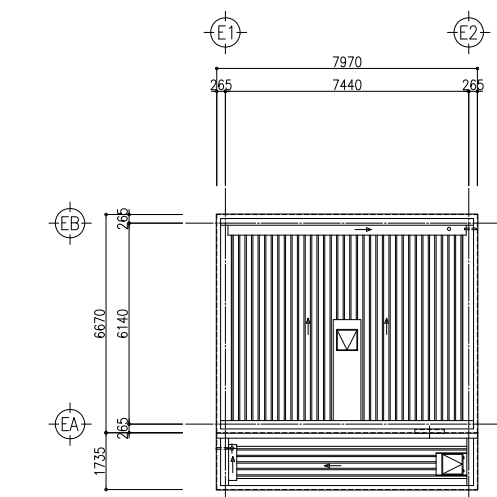
屋根伏図
