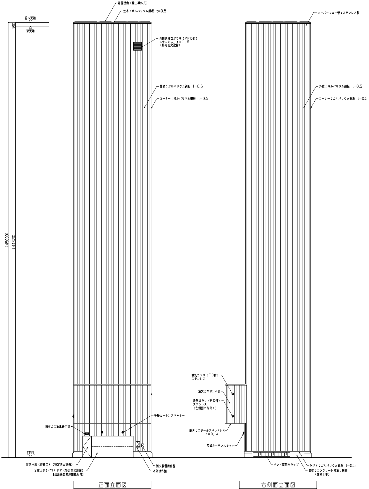
正面立面図
