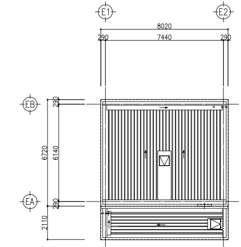
屋根伏図
