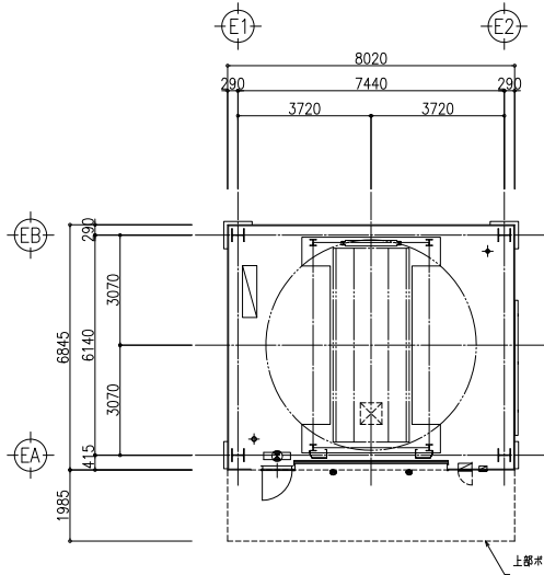
平面配置図
