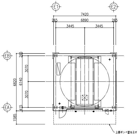
平面配置図
