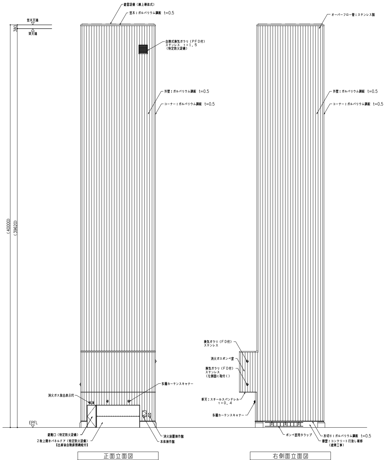
正面立面図
