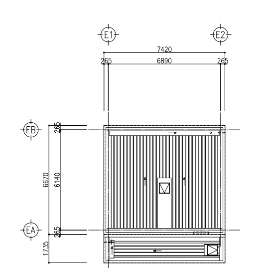
屋根伏図
