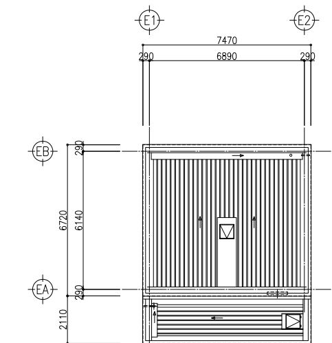
屋根伏図
