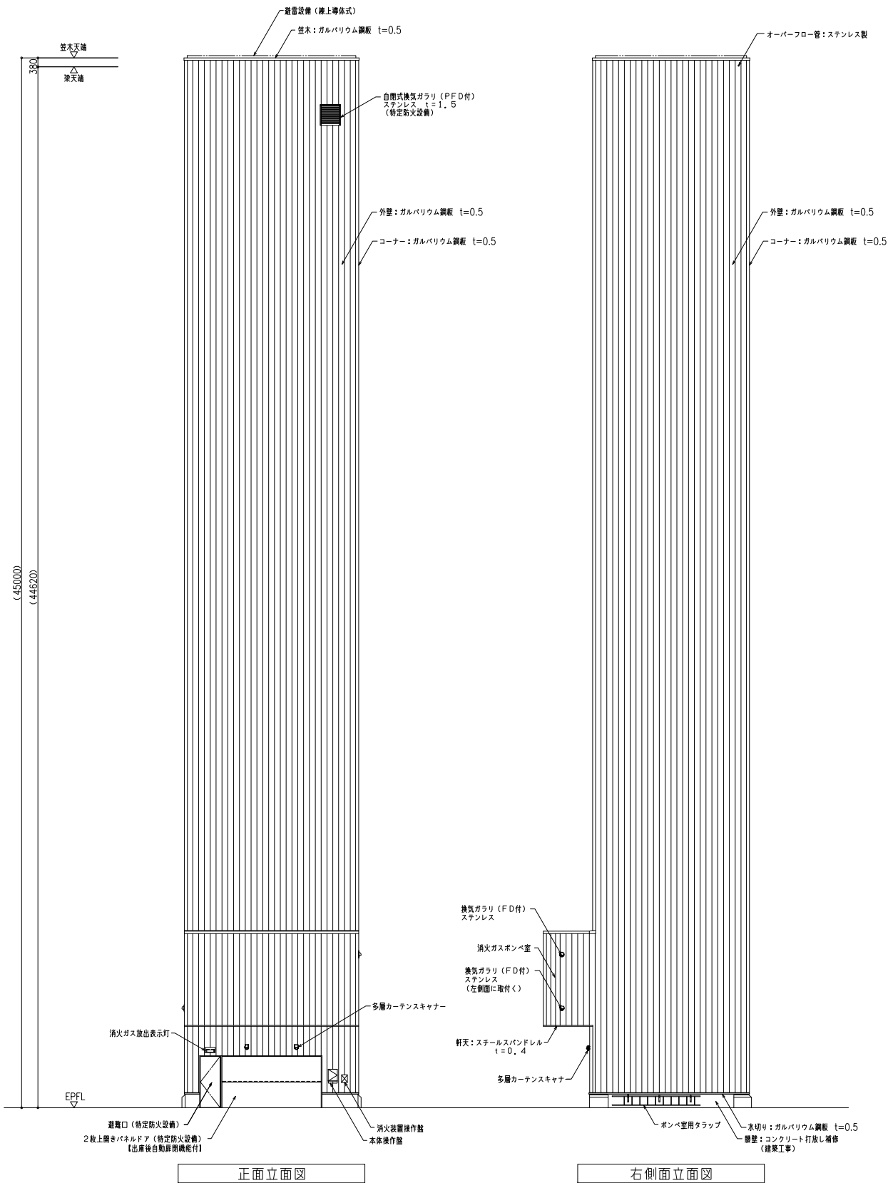
正面立面図
