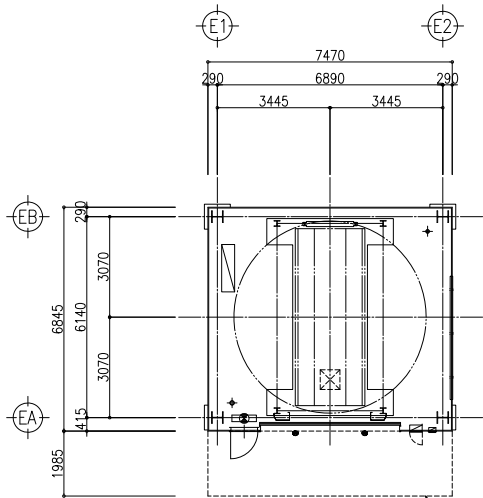
平面配置図
