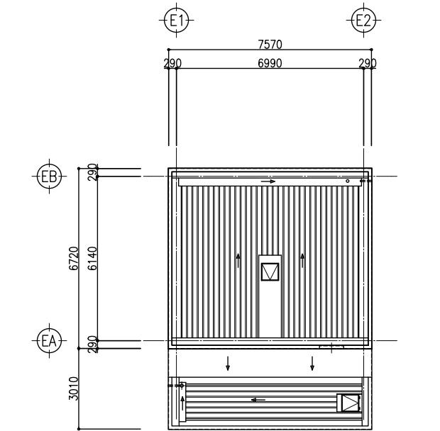
屋根伏図
