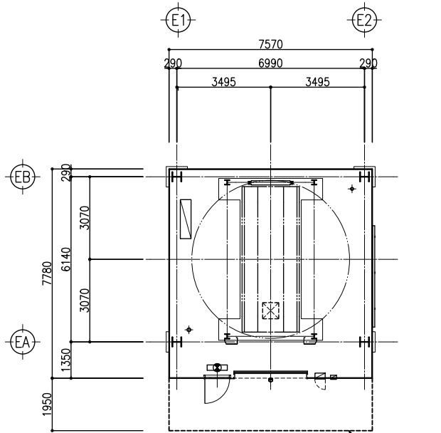
平面配置図
