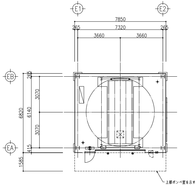
平面配置図
