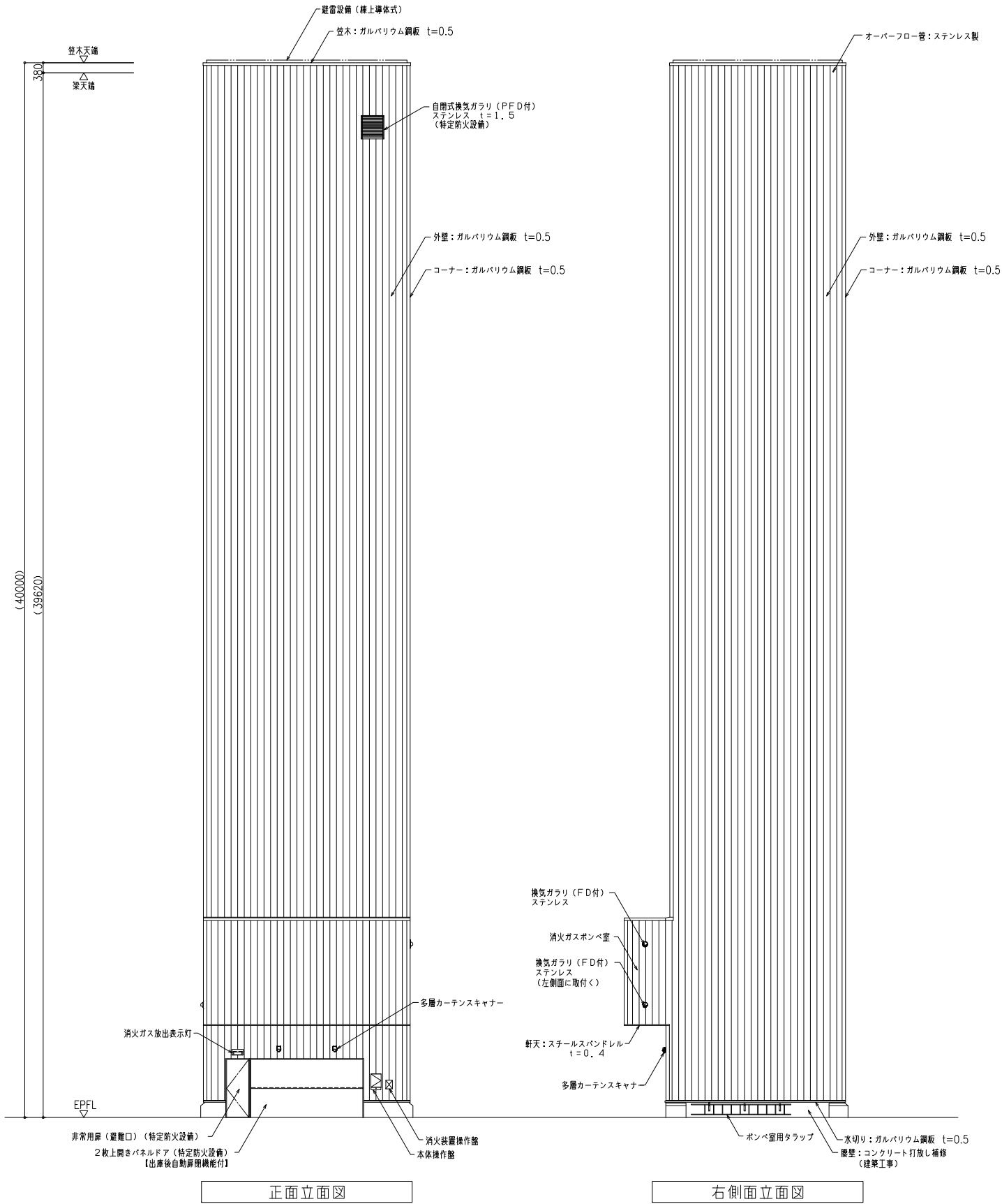
正面立面図
