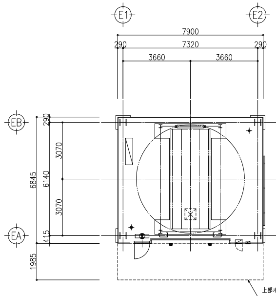
平面配置図
