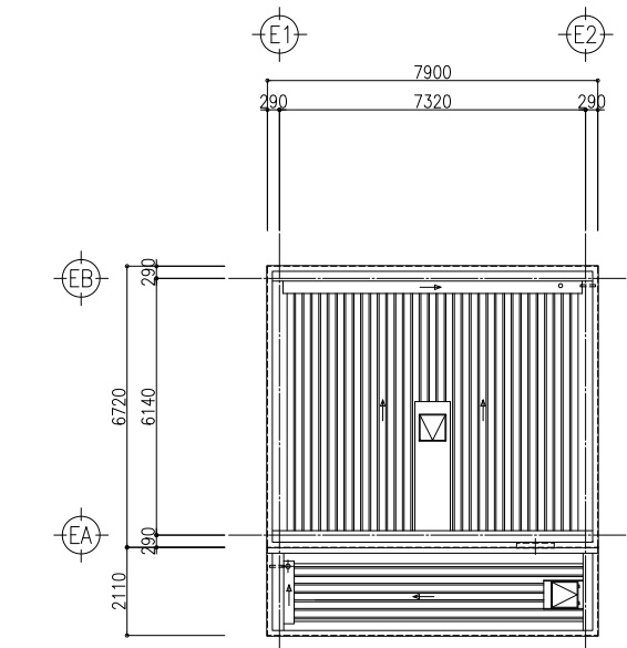
屋根伏図
