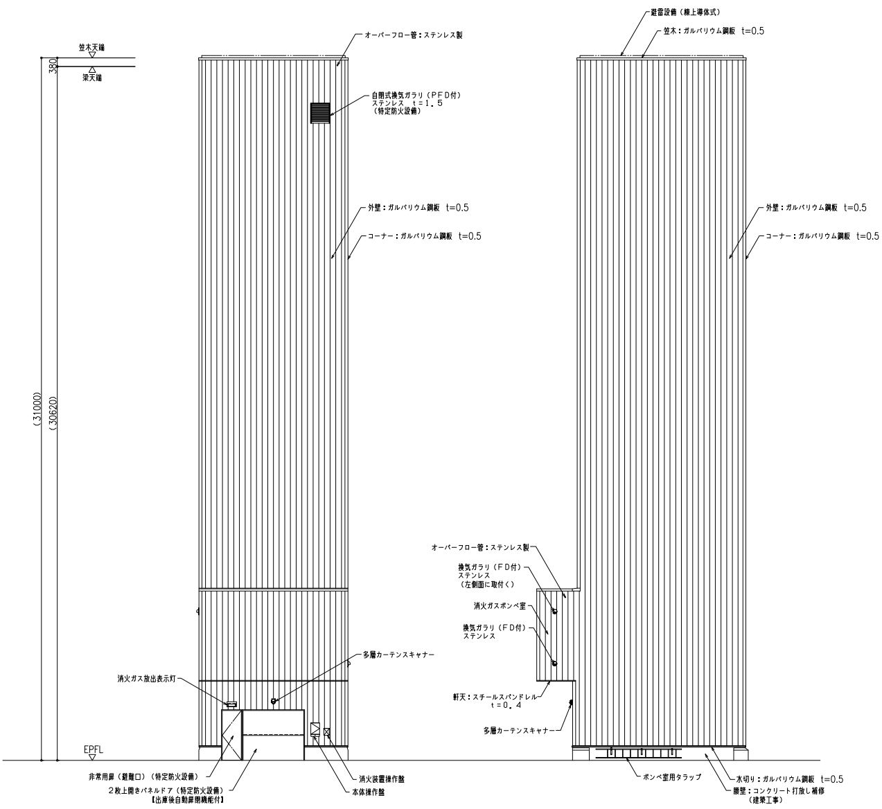
正面立面図
