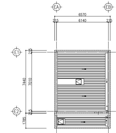
屋根伏図
