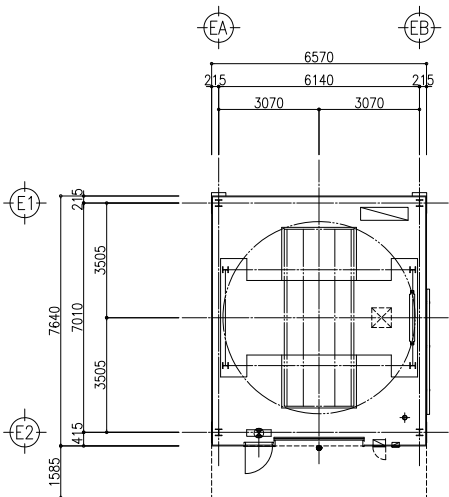
平面配置図
