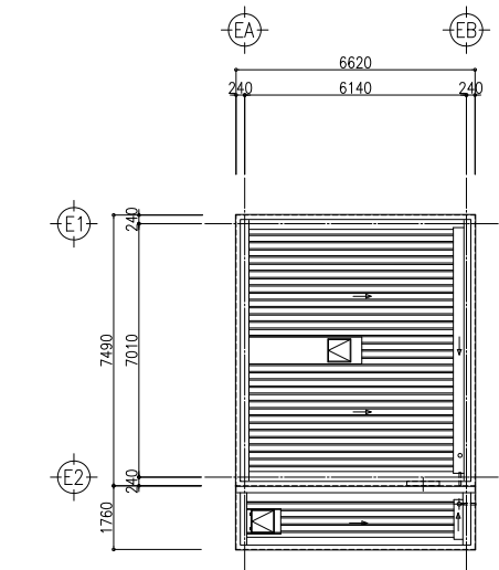
屋根伏図
