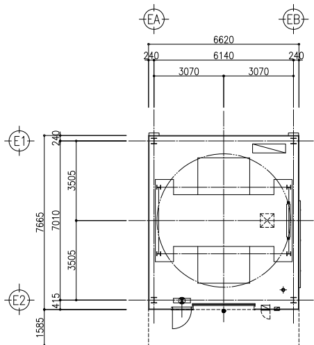
平面配置図
