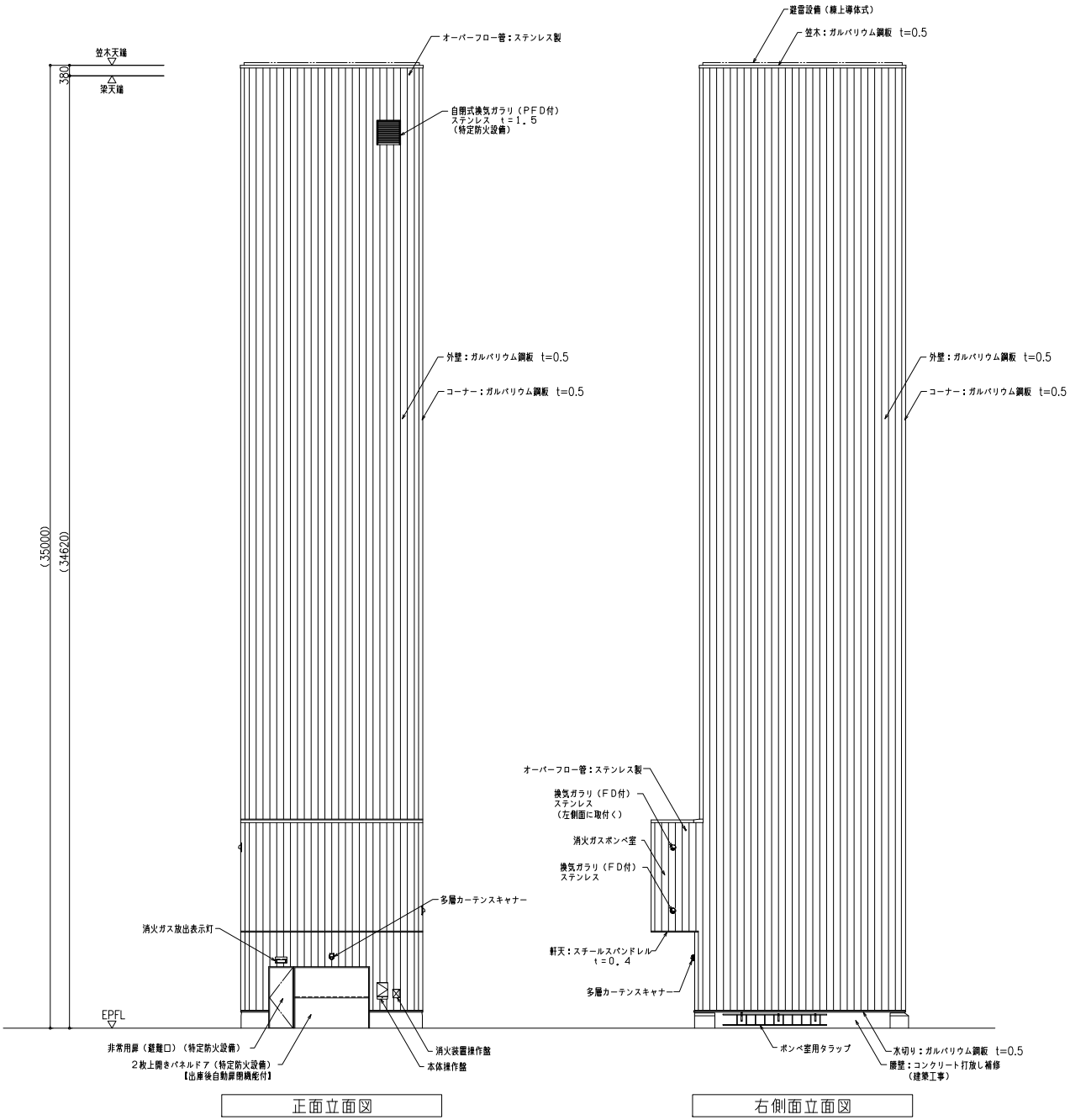
正面立面図
