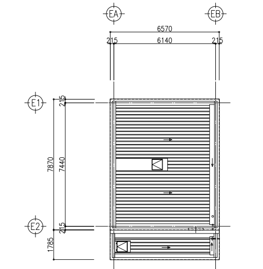
屋根伏図
