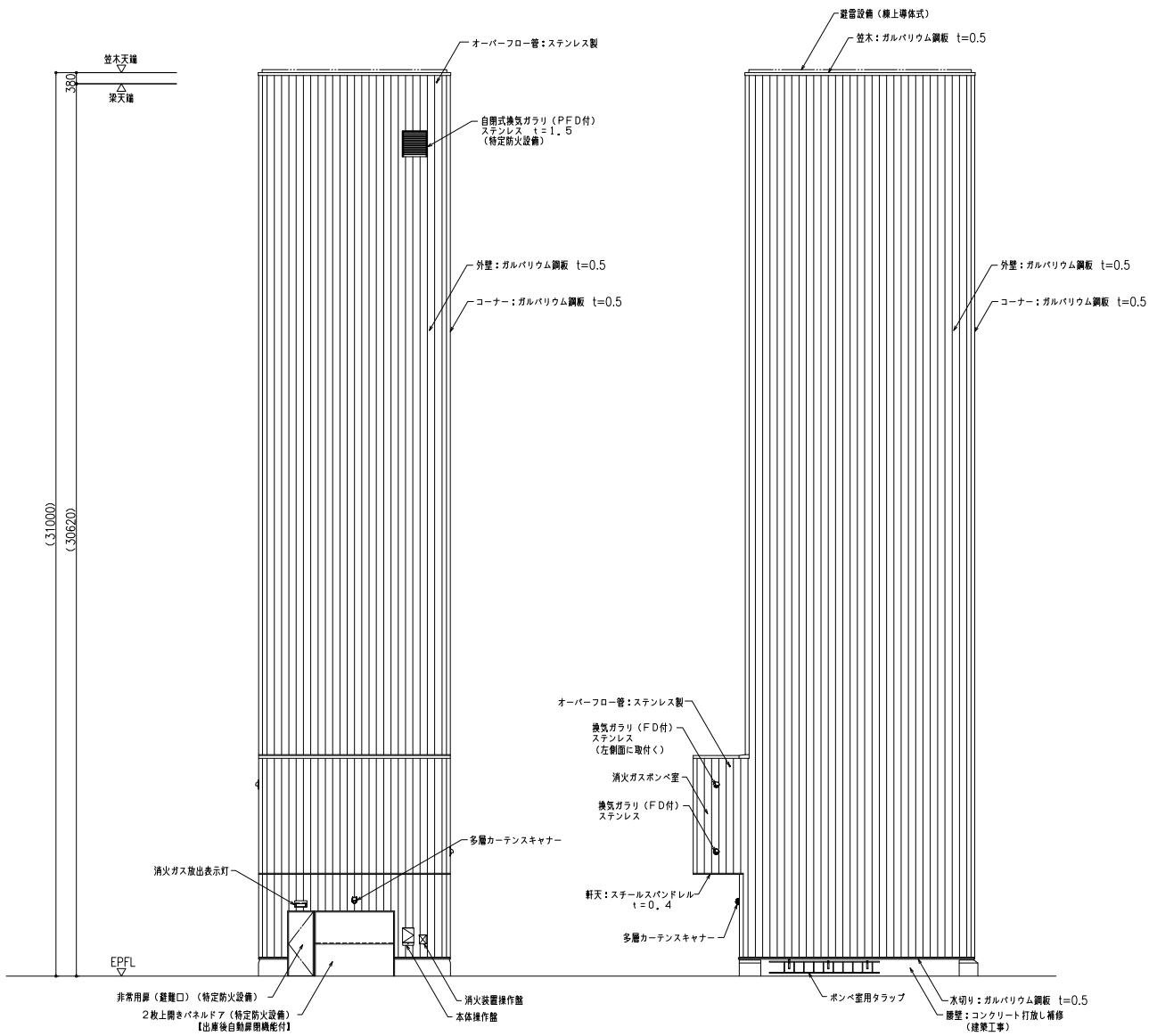
正面立面図
