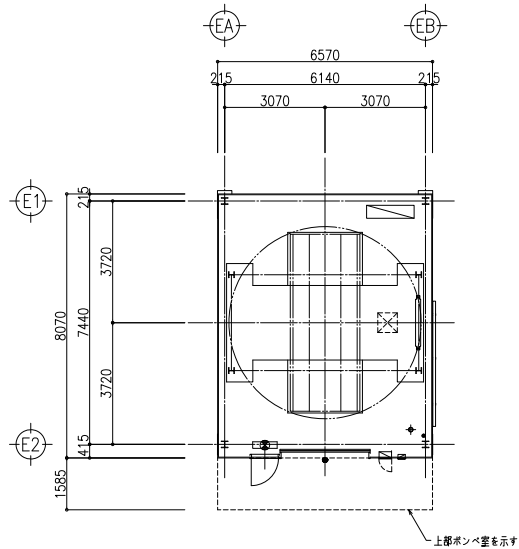
平面配置図
