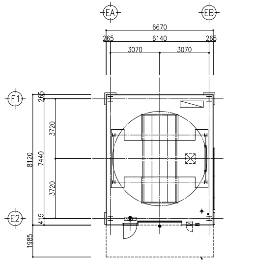
平面配置図
