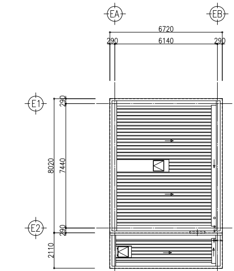
屋根伏図
