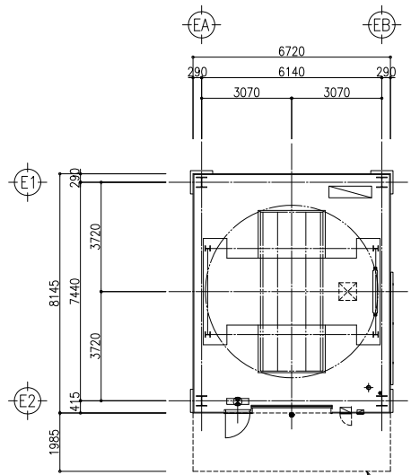
平面配置図
