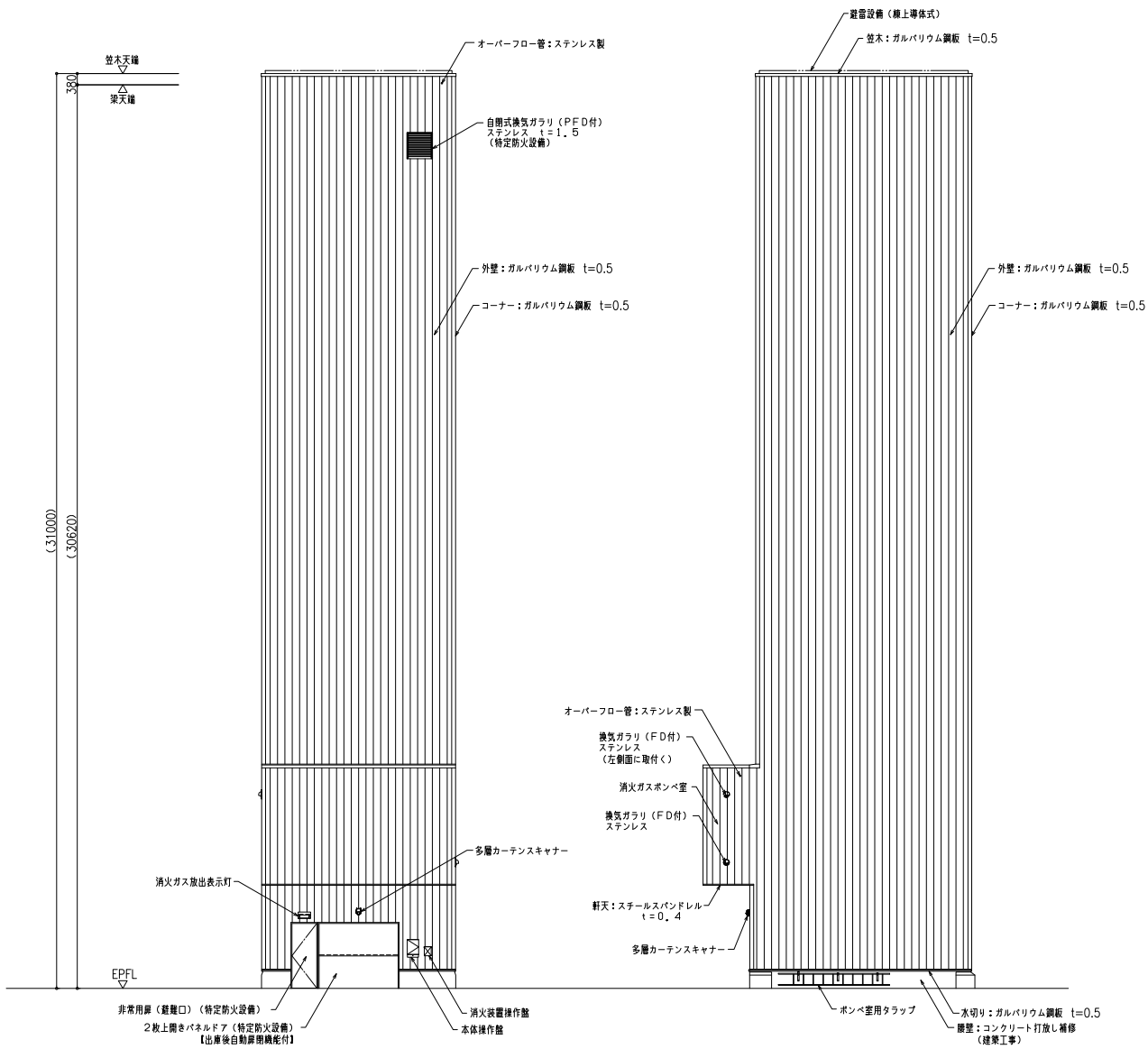
正面立面図
