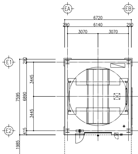
平面配置図
