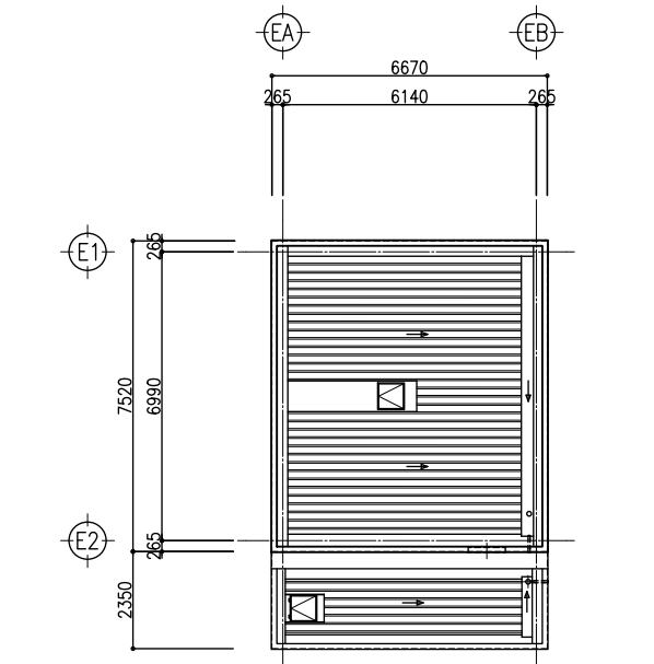
屋根伏図
