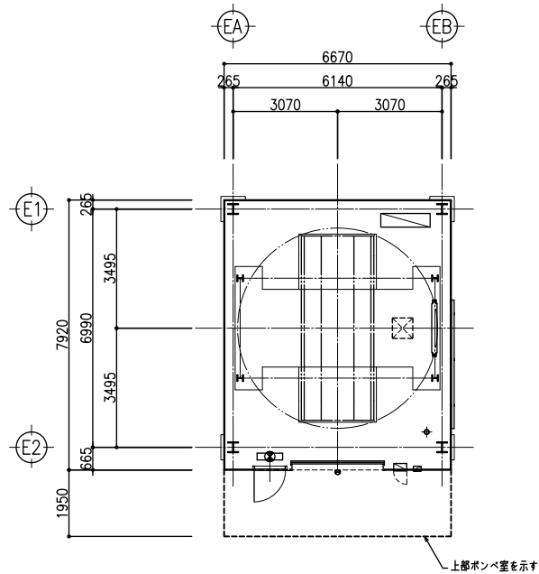
平面配置図
