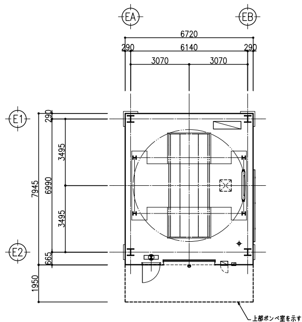
平面配置図
