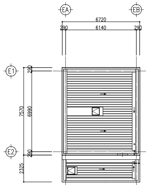
屋根伏図
