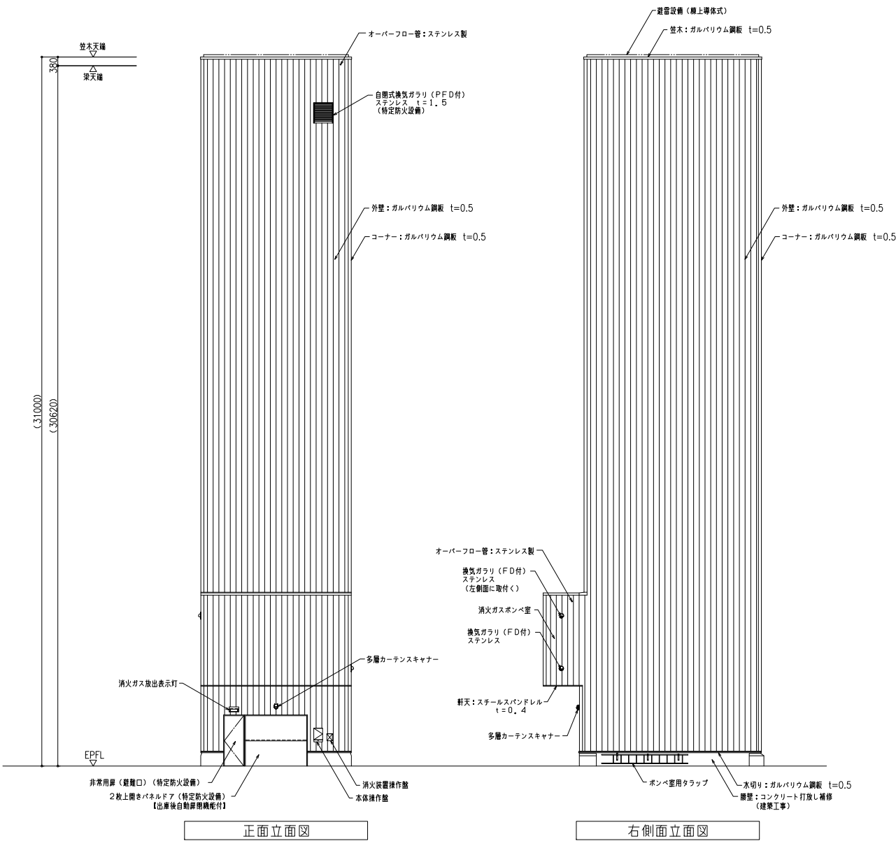
正面立面図
