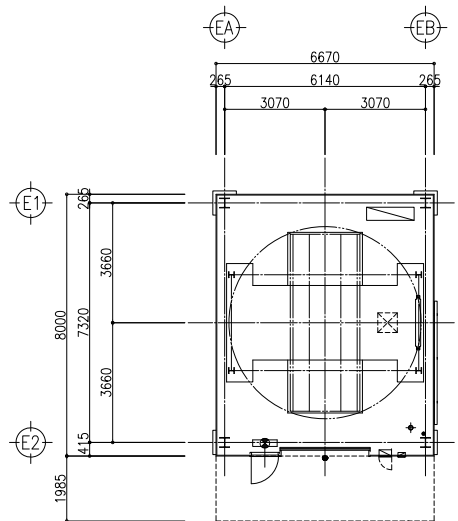
平面配置図
