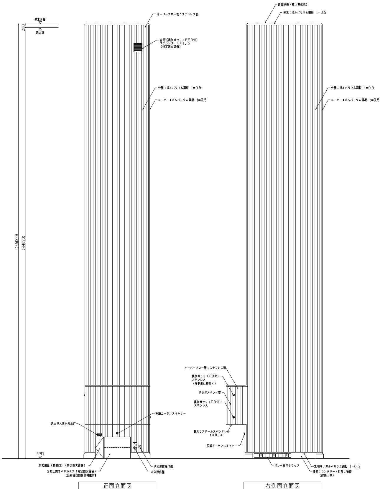
正面立面図
