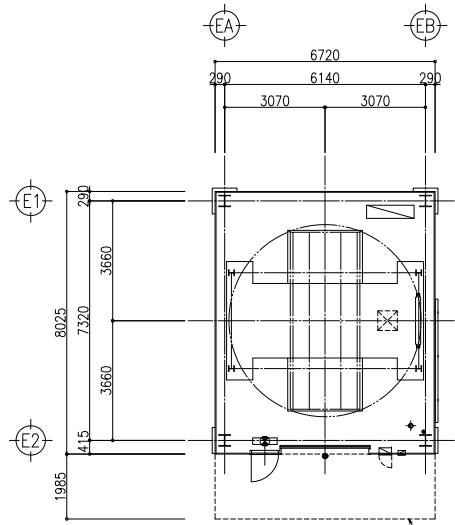
平面配置図
