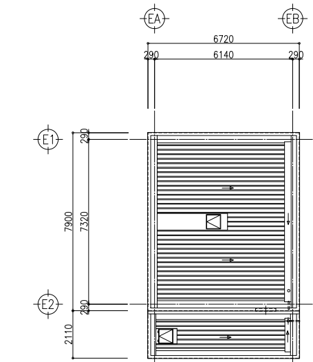
屋根伏図
