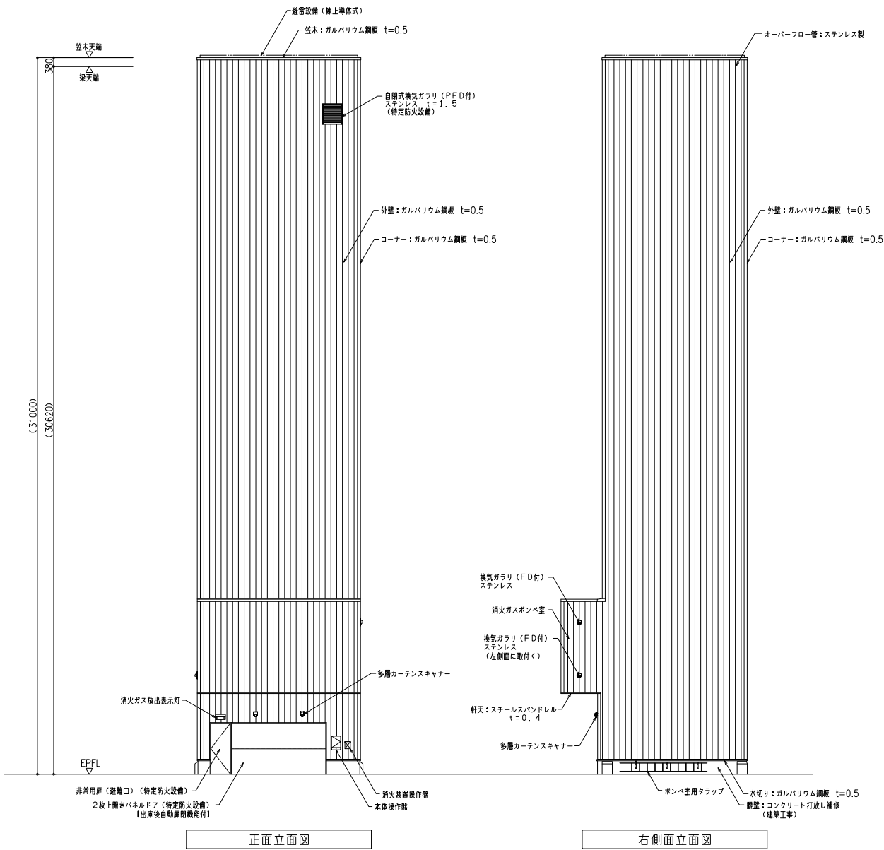
正面立面図
