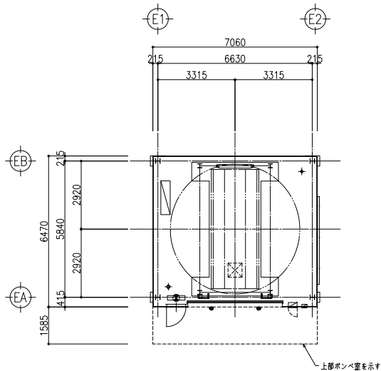
平面配置図
