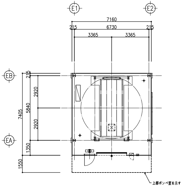
平面配置図
