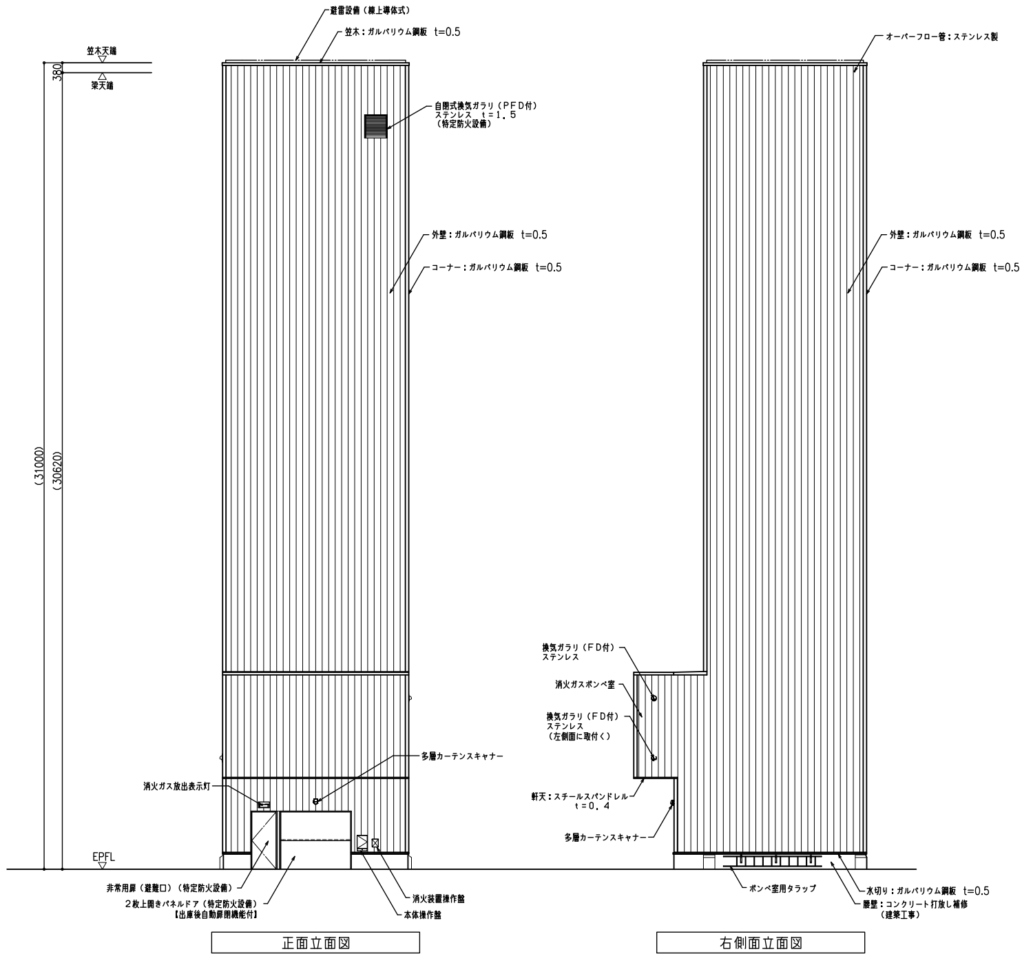
正面立面図
