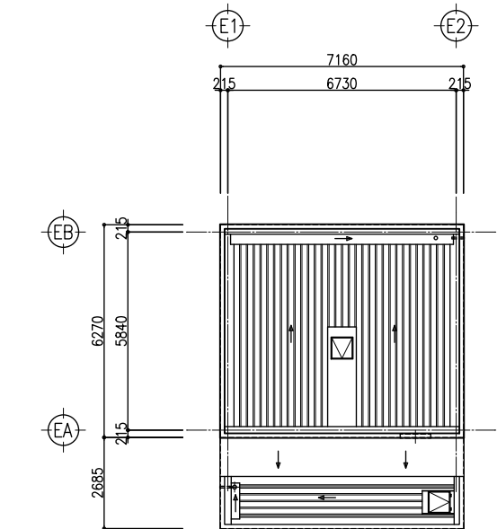
屋根伏図
