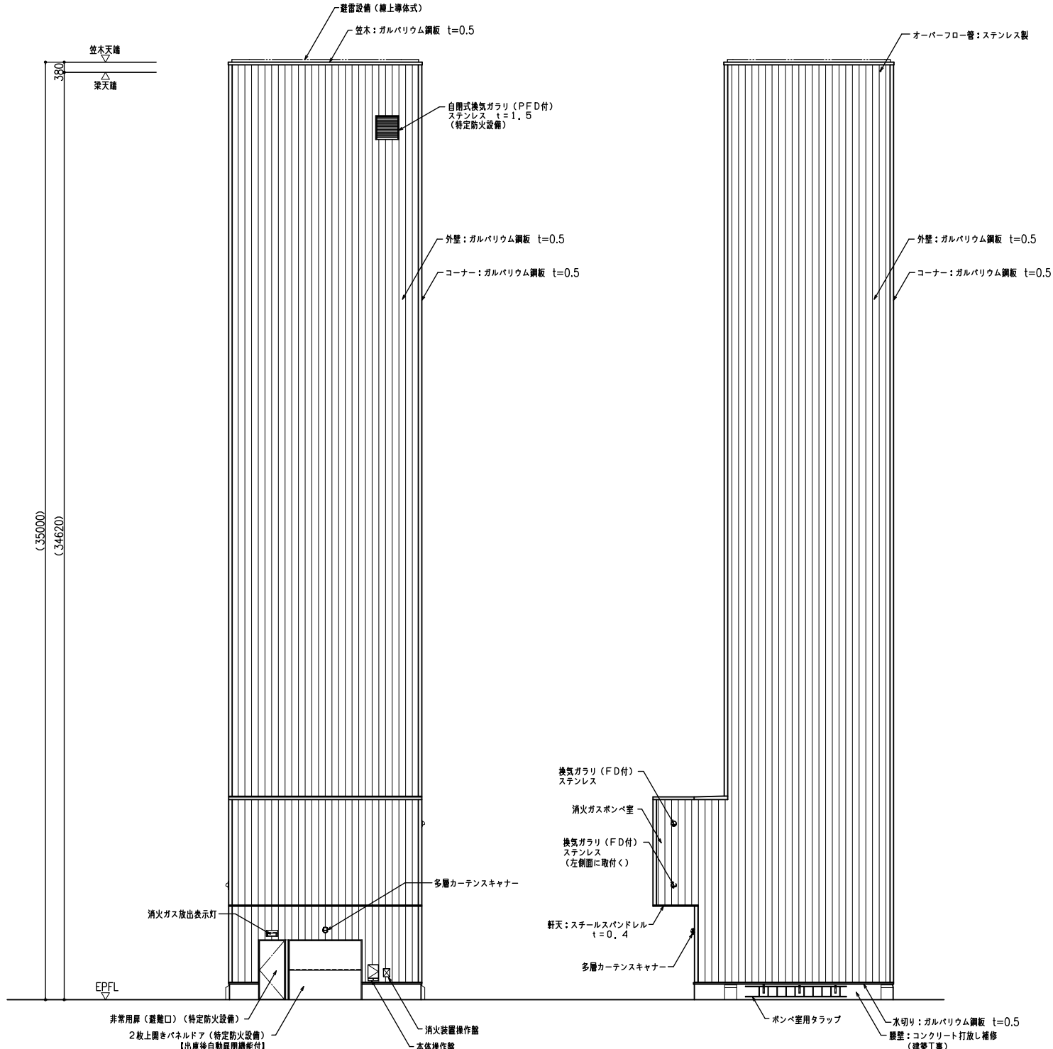
正面立面図
