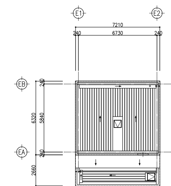
屋根伏図
