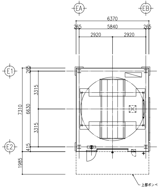
平面配置図
