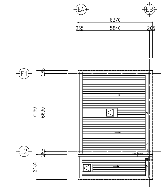
屋根伏図
