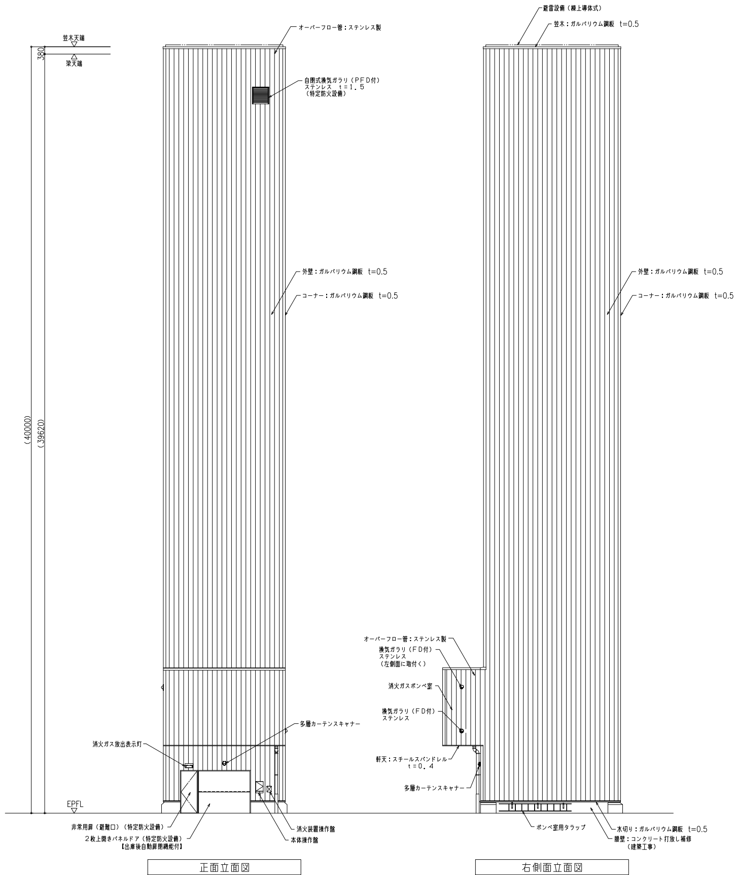
正面立面図
