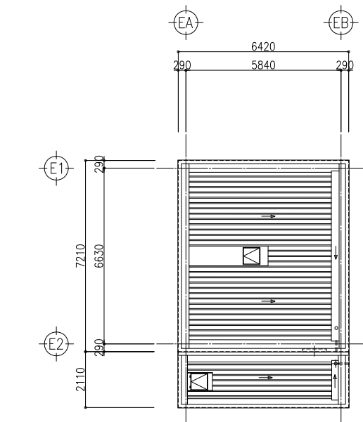
屋根伏図
