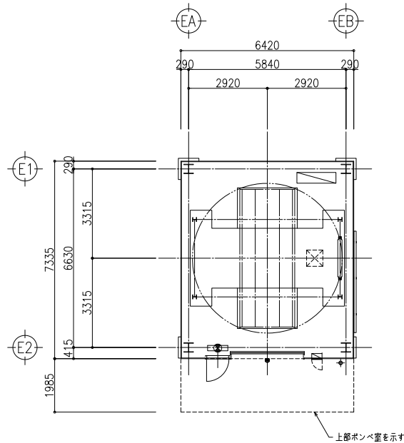
平面配置図
