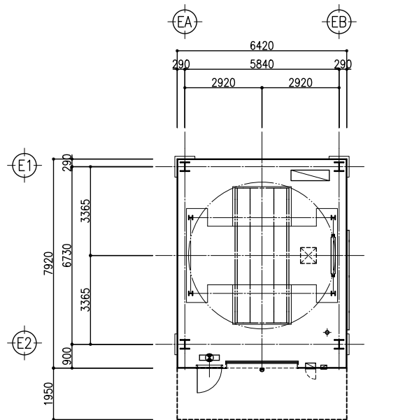
平面配置図
