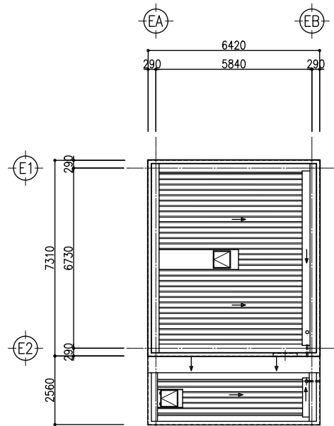
屋根伏凶
